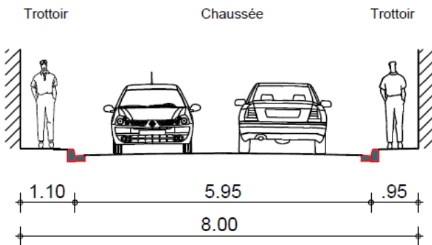
Profil en travers existant
