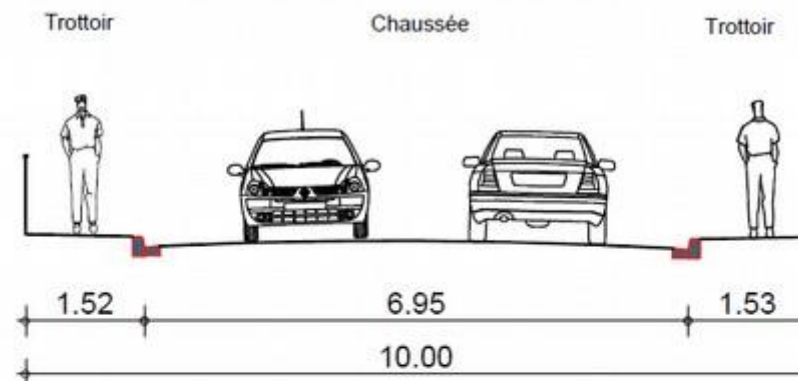
Profil en travers existant
