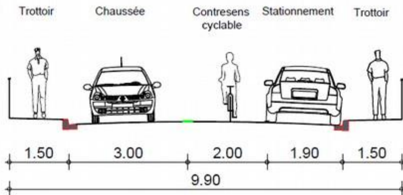
Profil en travers temporaire
