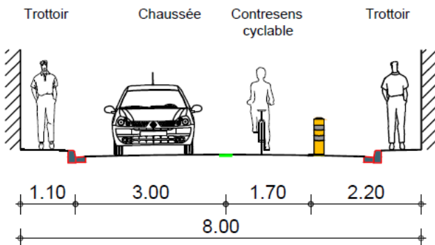
Profil en travers temporaire
